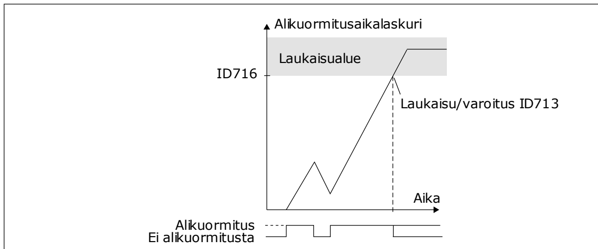
Kuva 60: Alikuormitusaikalaskurin toiminta
