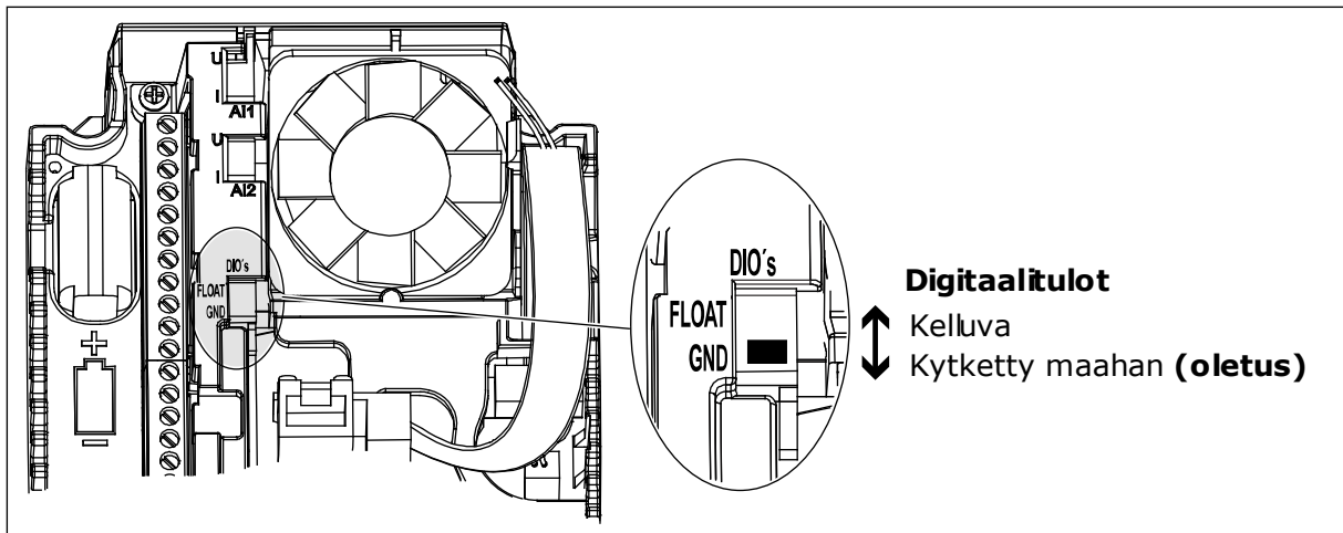
Kuva 9: DIP-kytkin
