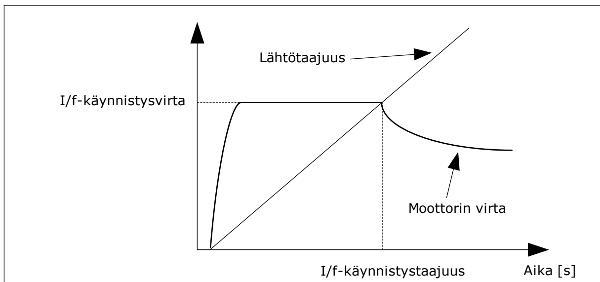
Kuva 25: I/f-käynnistysten parametrit
