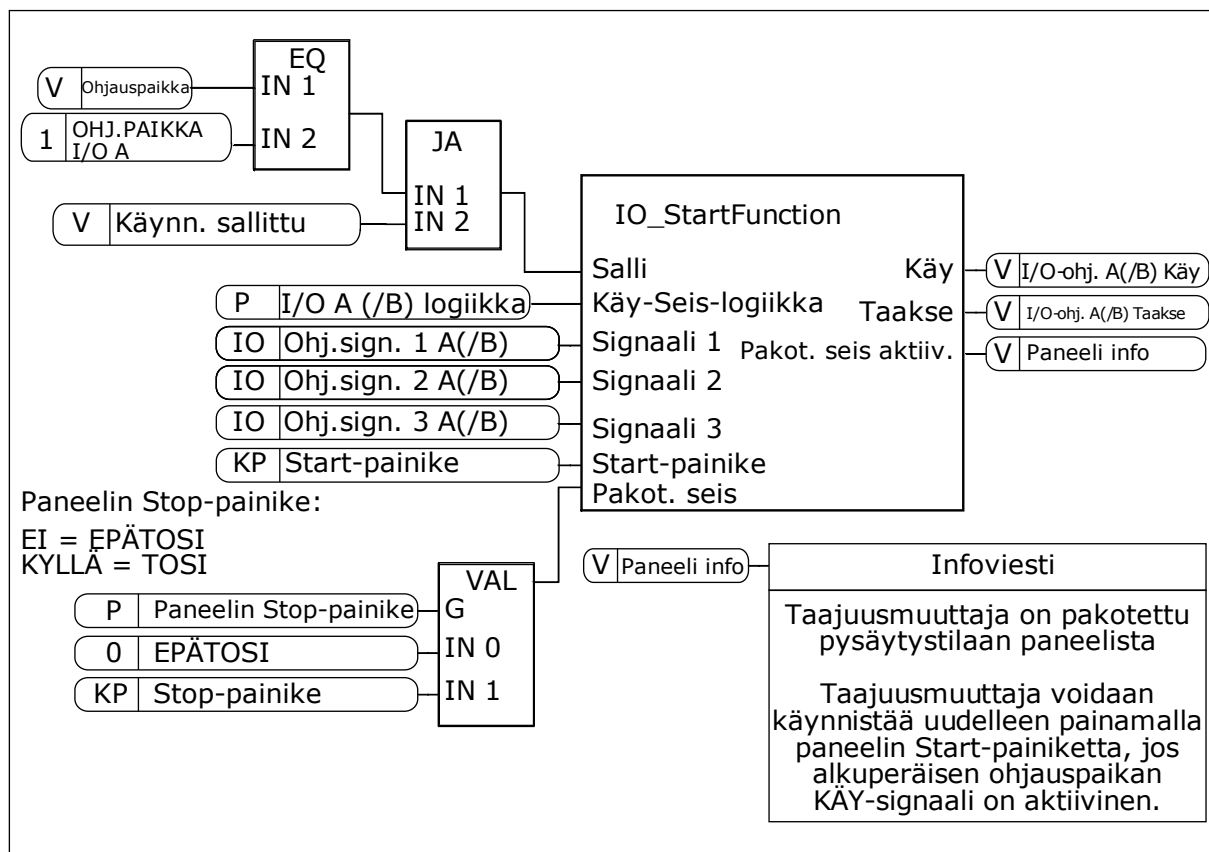
Kuva 27: I/O A Käy/Seis -logiikan lohkokaaavio.
