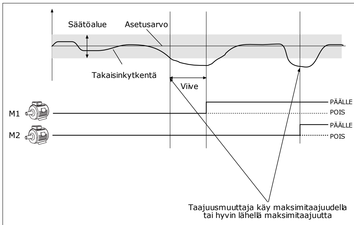
Kuva 79: Monipumpputoiminto
