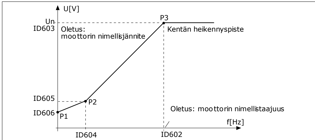
Kuva 24: Ohjelmoitava U/f-käyrä
