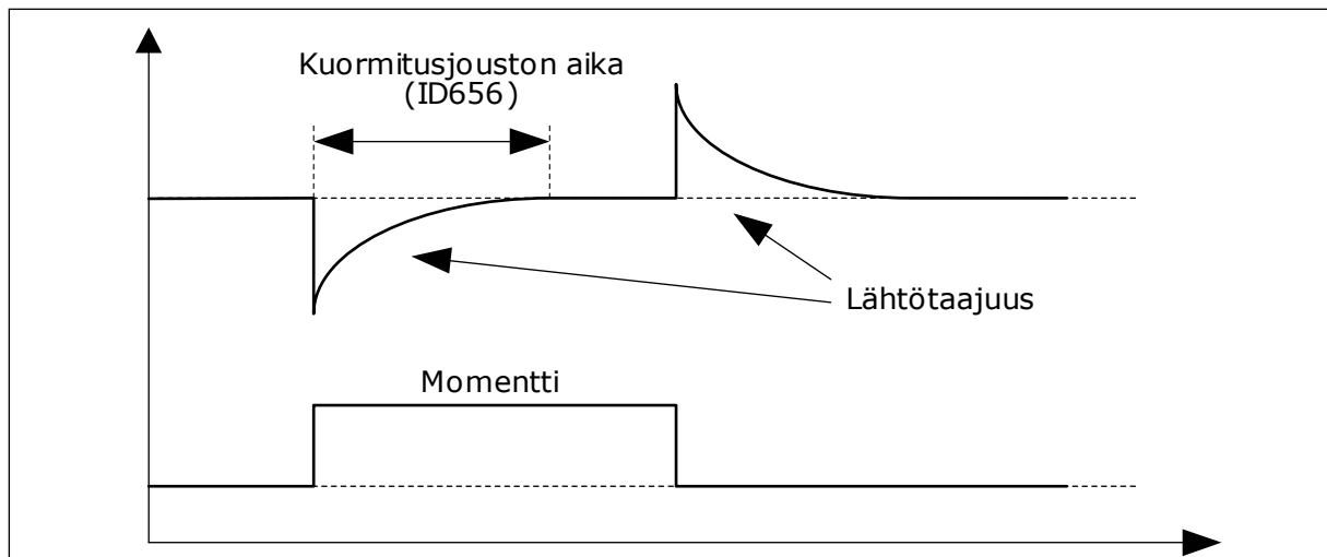
Kuva 21: Kuormitusjoustotoiminto
