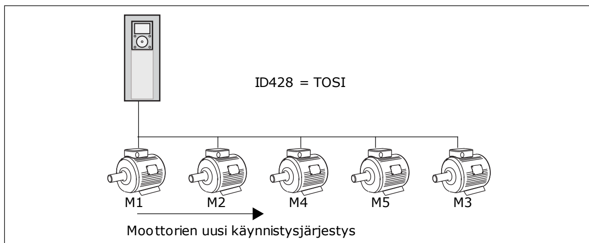
Kuva 82: Lukituslogiikka 3
