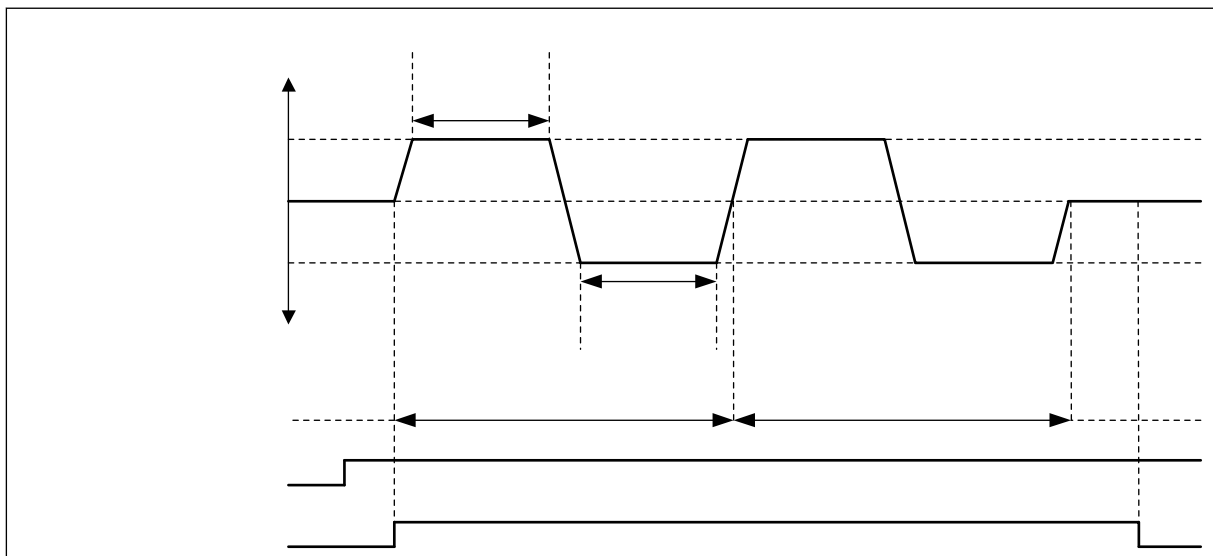
Kuva 90: Automaattinen puhdistustoiminto
