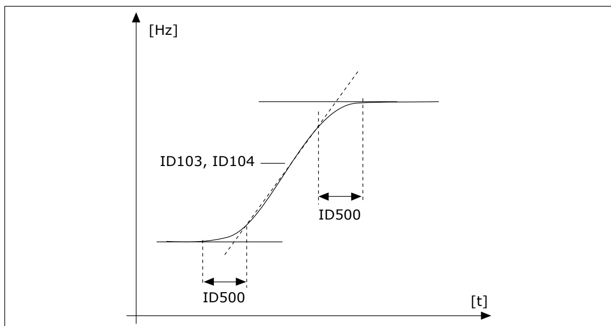
Kuva 40: Kiihdytys-/hidastuskäyrä (S-muoto)
