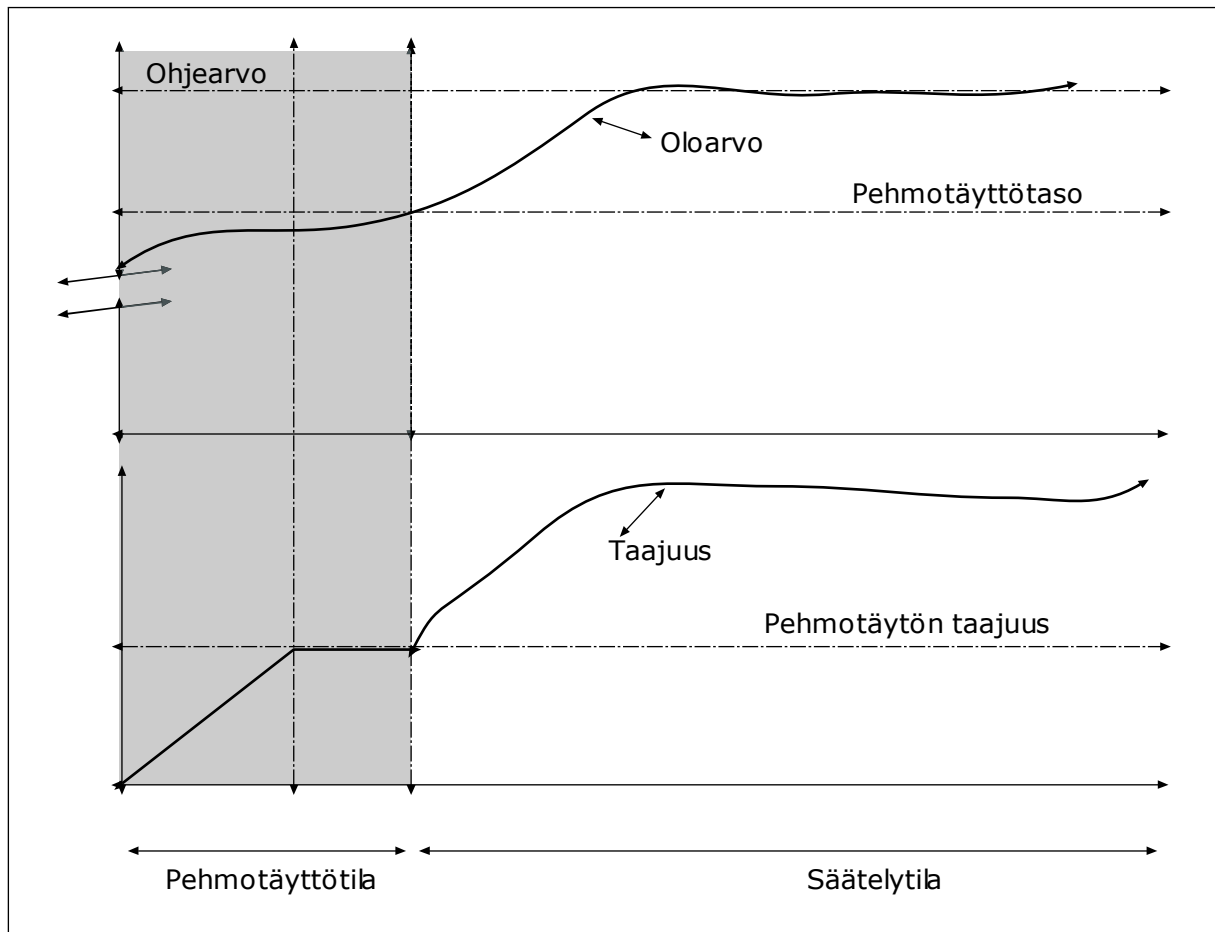
Kuva 76: Pehmotäyttötoiminto
