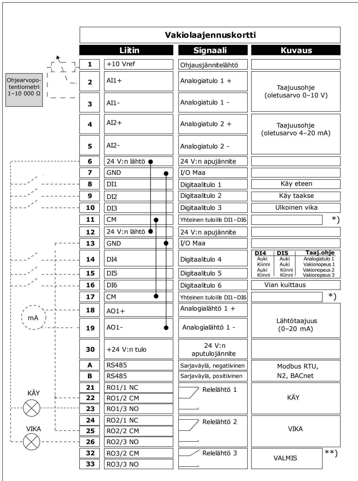
Kuva 4: Vakiosovelluksen oletusohjausliitännät
