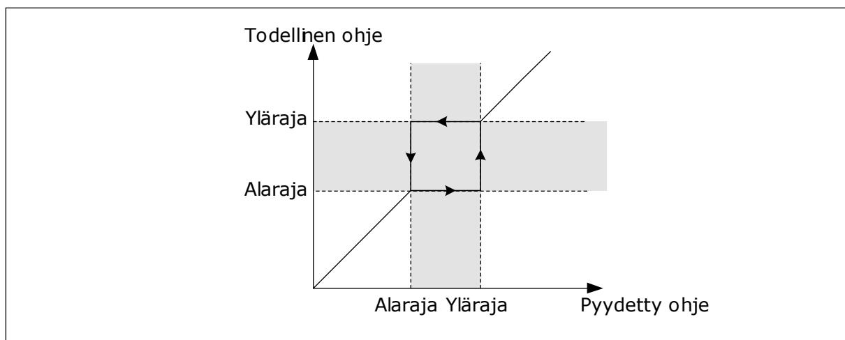
Kuva 53: Estetyt taajuudet
