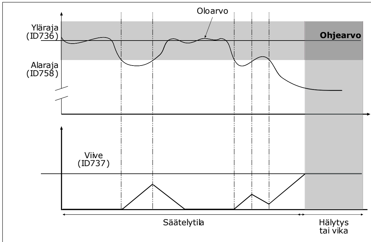
Kuva 73: Takaisinkytkennän valvontatoiminto
